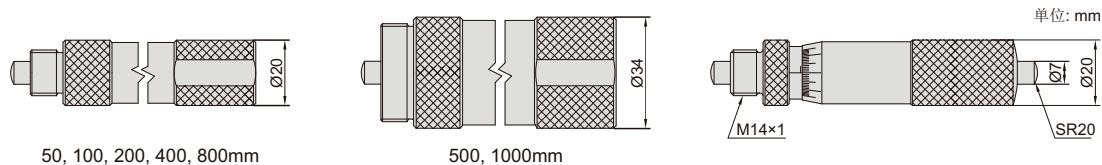
延长杆隔热
